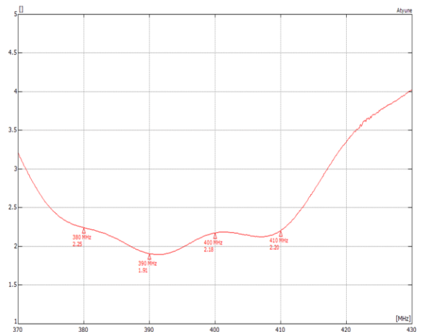
VSWR*
