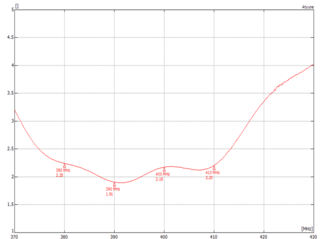
VSWR*
