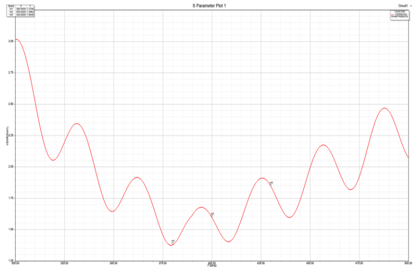
VSWR*
