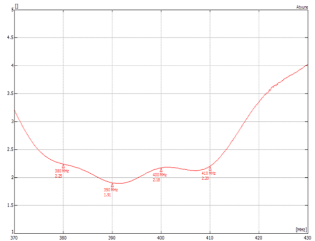
VSWR*
