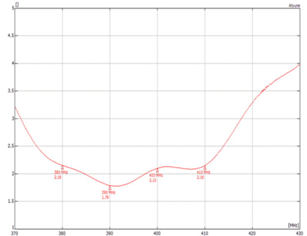
VSWR*
