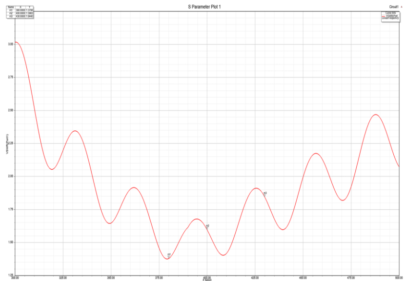
VSWR*
