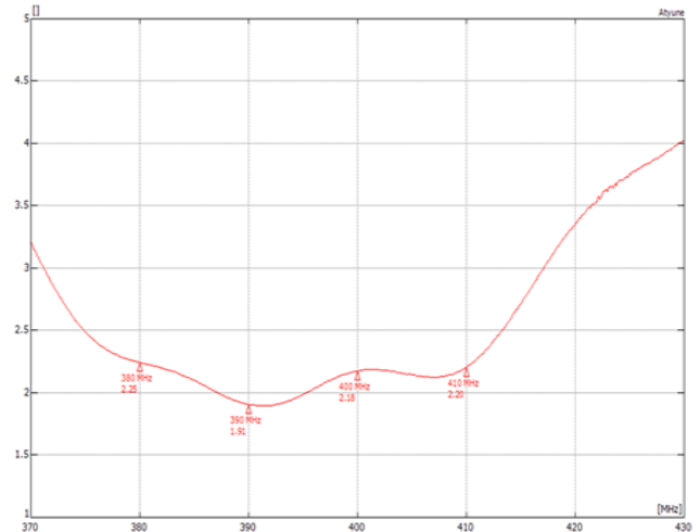
VSWR*
