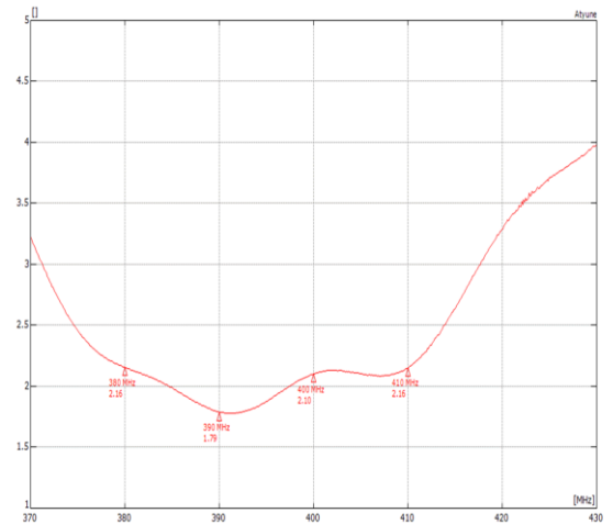
VSWR*
