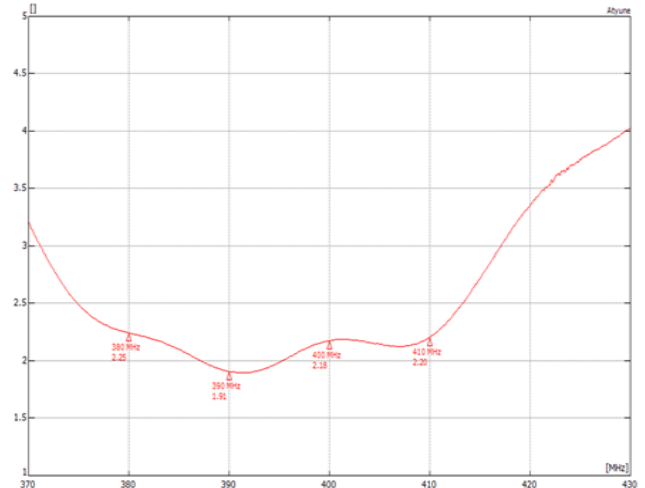
VSWR*
