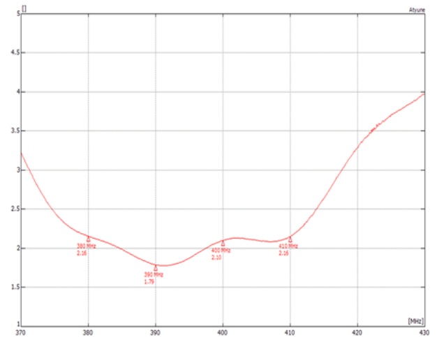
VSWR*
