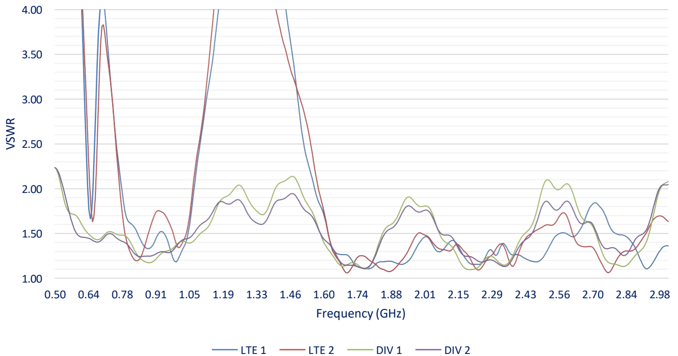
LTE VSWR
