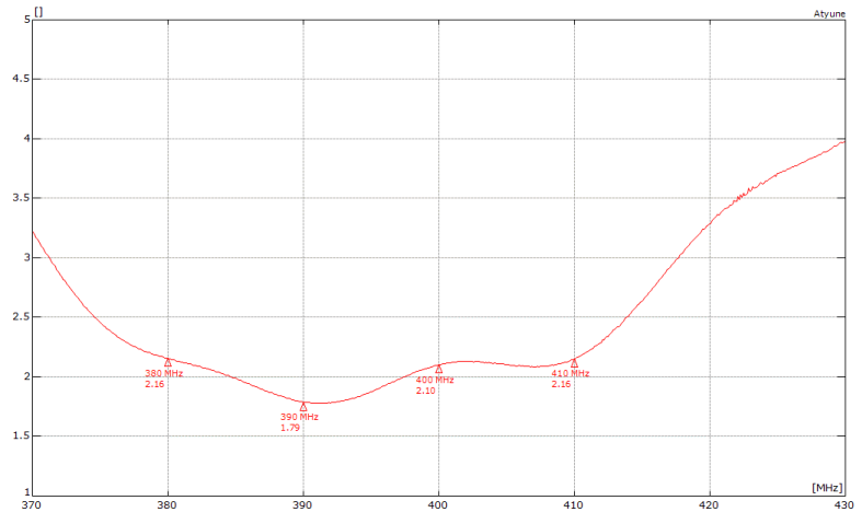
VSWR*
