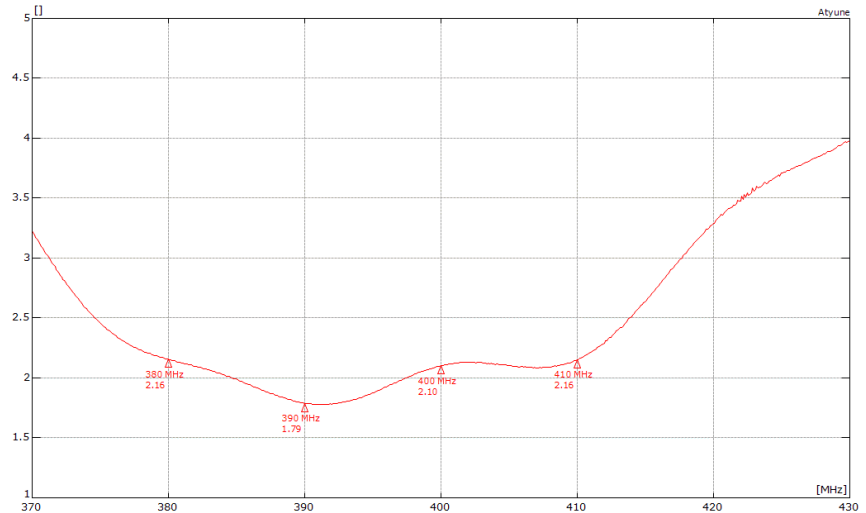
VSWR*
