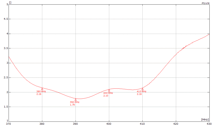
VSWR*
