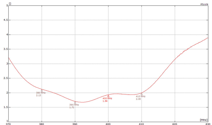
VSWR*
