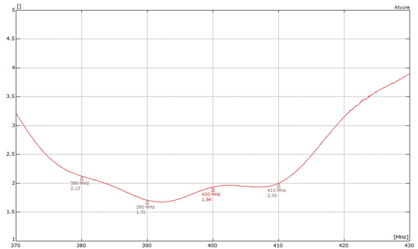
VSWR*
