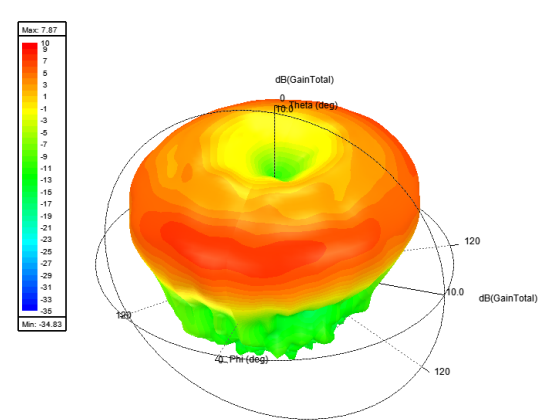
3600MHz
