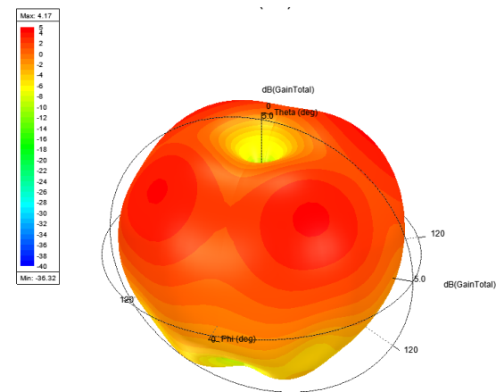
2140MHz
