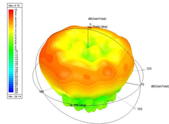
2600MHz
