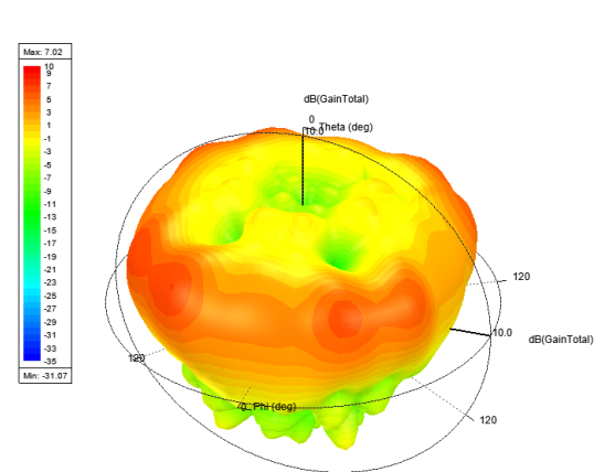
2140MHz
