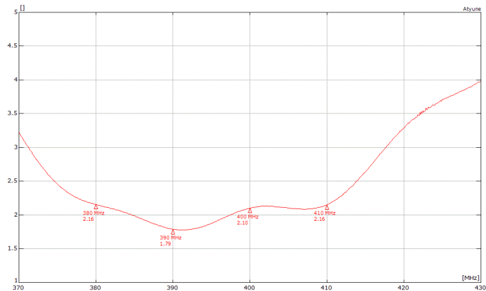
VSWR*
