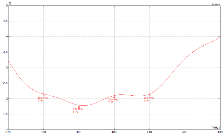
VSWR*
