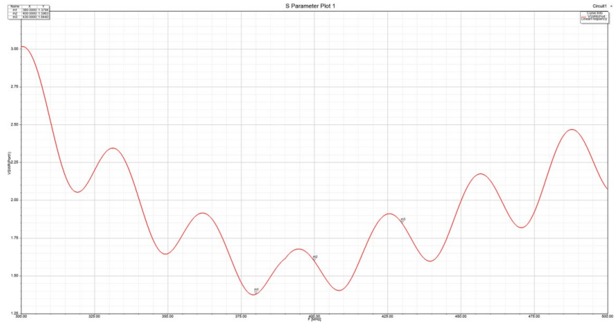
VSWR*
