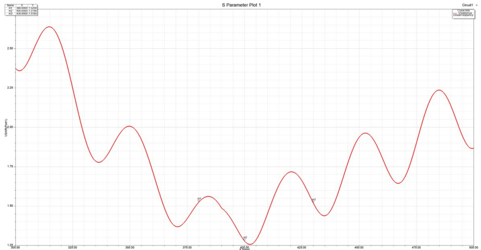
VSWR*
