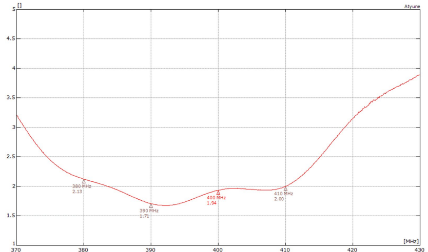
VSWR*
