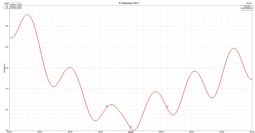
VSWR*
