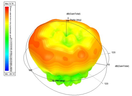
2600MHz
