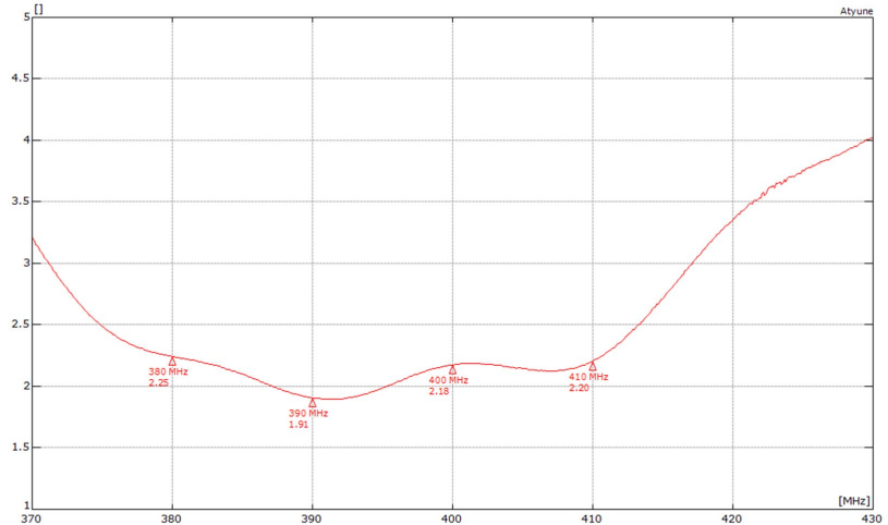
VSWR*
