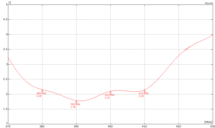
VSWR*
