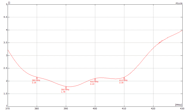
VSWR*
