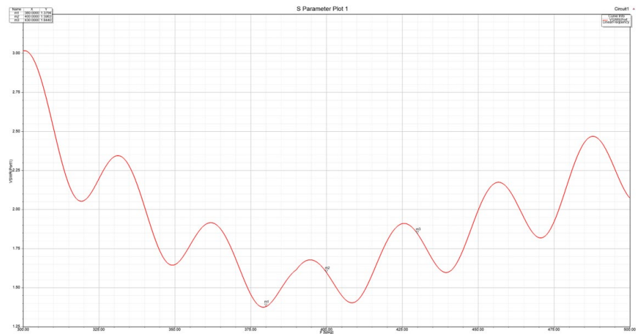
VSWR*
