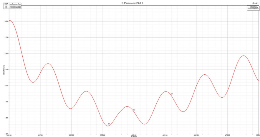
VSWR*
