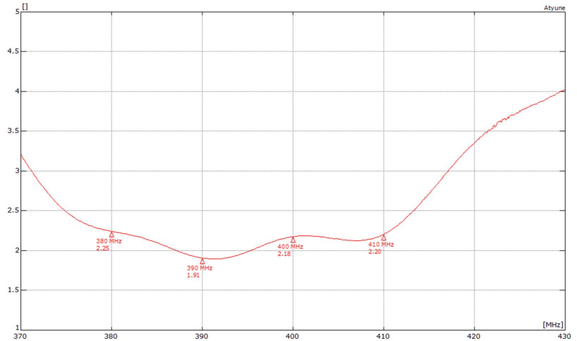
VSWR*
