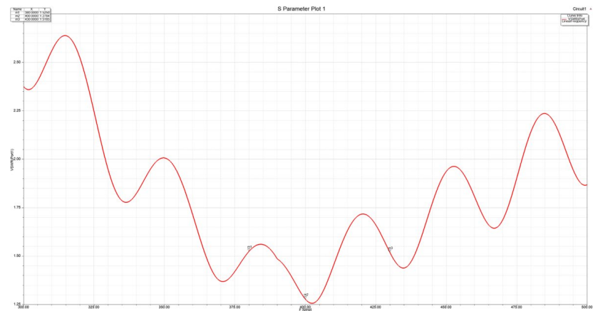
VSWR*
