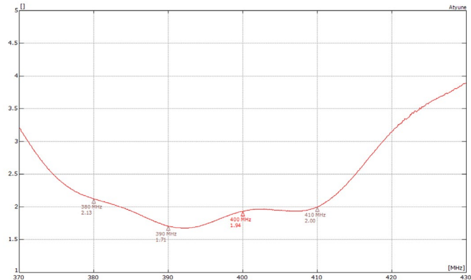
VSWR*
