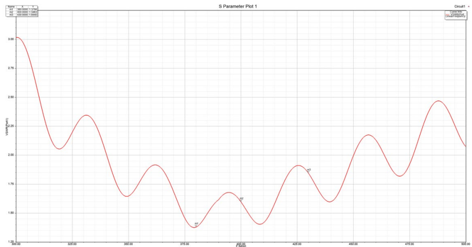
VSWR*
