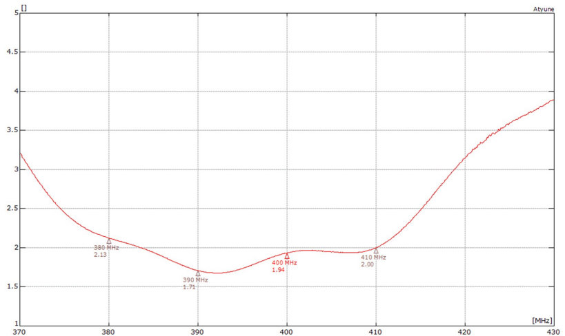
VSWR*
